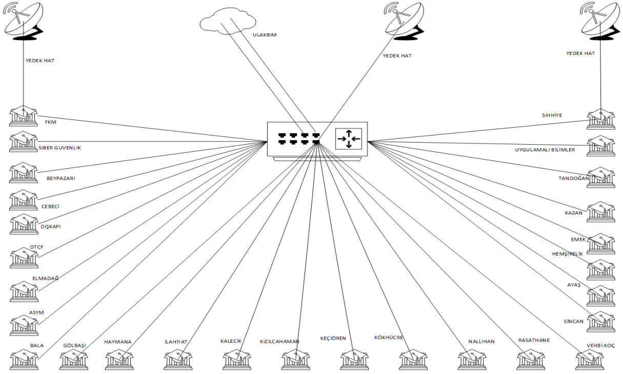
Şekil-3: Ankara Üniversitesi Ağ Topolojisi
